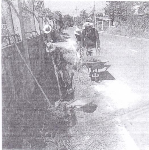
ภาพถ่ายการดำเนินงานธนาคารน้ำใต้ดินภายในบริเวณบ้านนอก หมู่ที่ ๑๐ จุดที่ ๗
